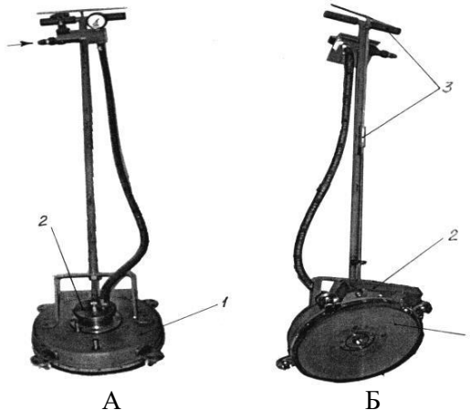
А – вид спереди: 1 – корпус; 2 – запорное устройство;
