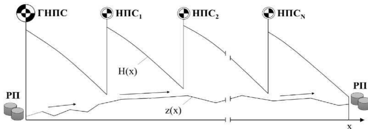
Рисунок 1 - Схема технологического участка нефтепровода
